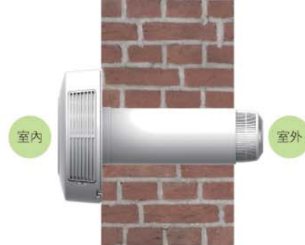
※ 牆面安裝示意圖
